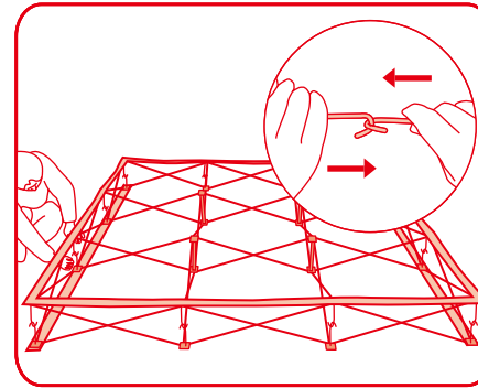
②上下左右の金具を留めます。(計16箇所) ※盤面を貼る側が上になるように注意してください。
