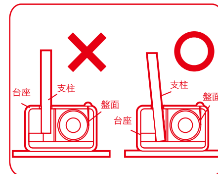
③支柱は奥までしっかりと差し込んでください。 ※斜めに差し込む事で、奥まで差し込む事が出来ません。
