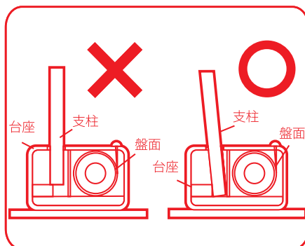
④支柱は奥までしっかりと差し込んでください。 ※斜めに差し込む事で、奥まで差し込む事が出来ません。
